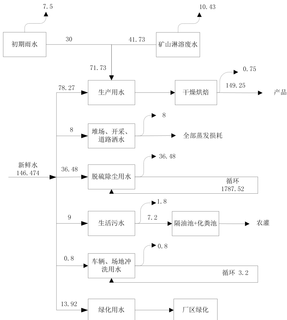
图1-5 项目用水平衡图 (单位: t/d)
