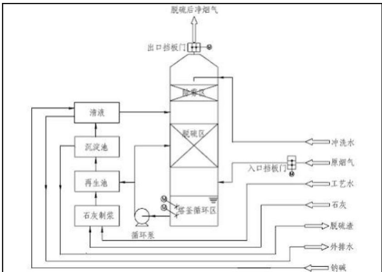
图 5-4 项目脱硫除尘工艺流程图
