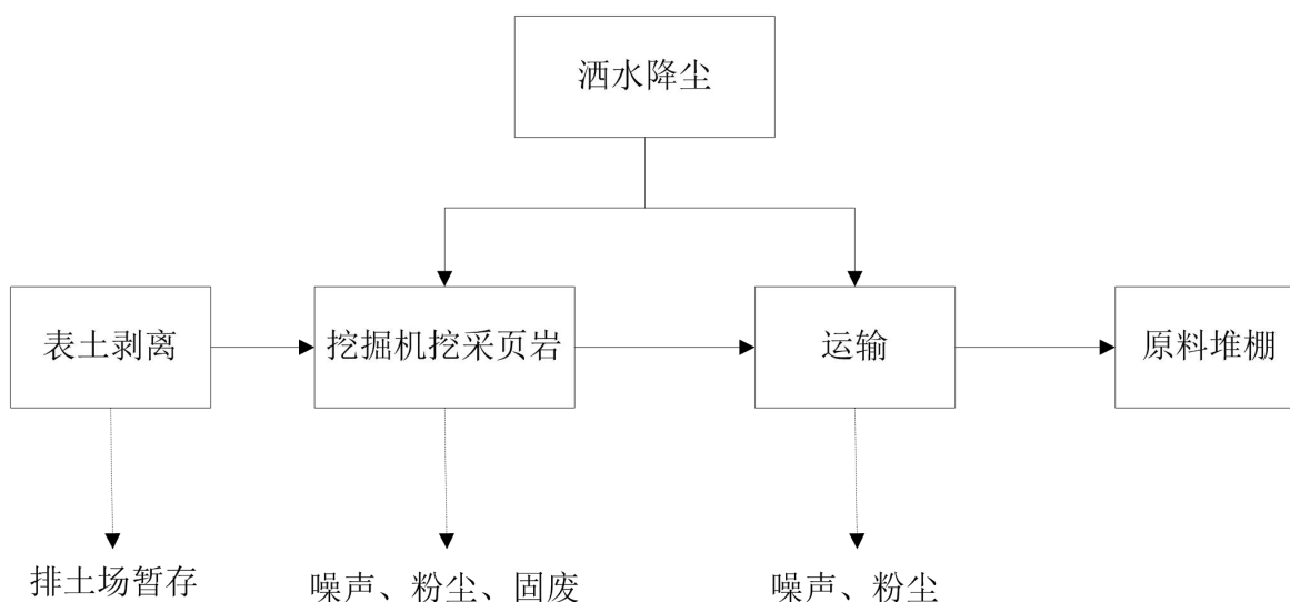
图 5-2 页岩开采工艺流程及产污环节图
