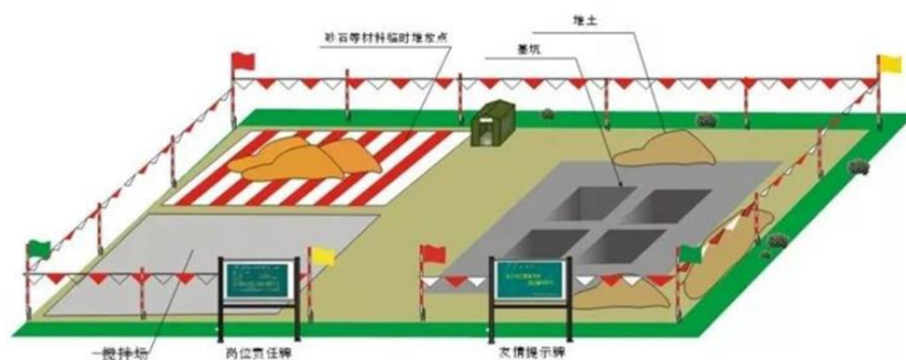
图 2-1 典型塔基施工平面布置示意图
