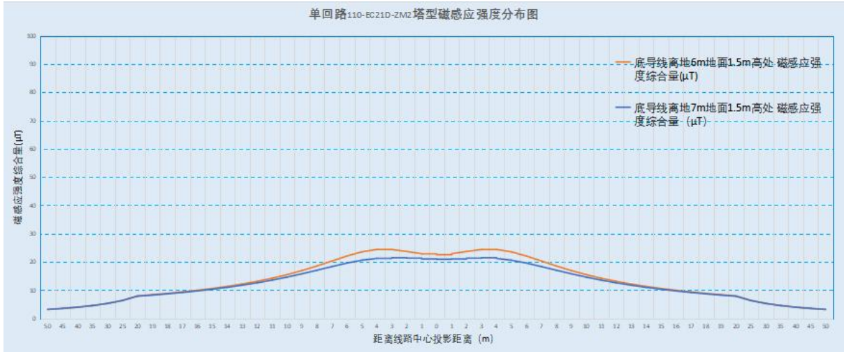
图 3-3 单回路 110-EC21D-ZM2 塔型工频磁感应强度分布图
