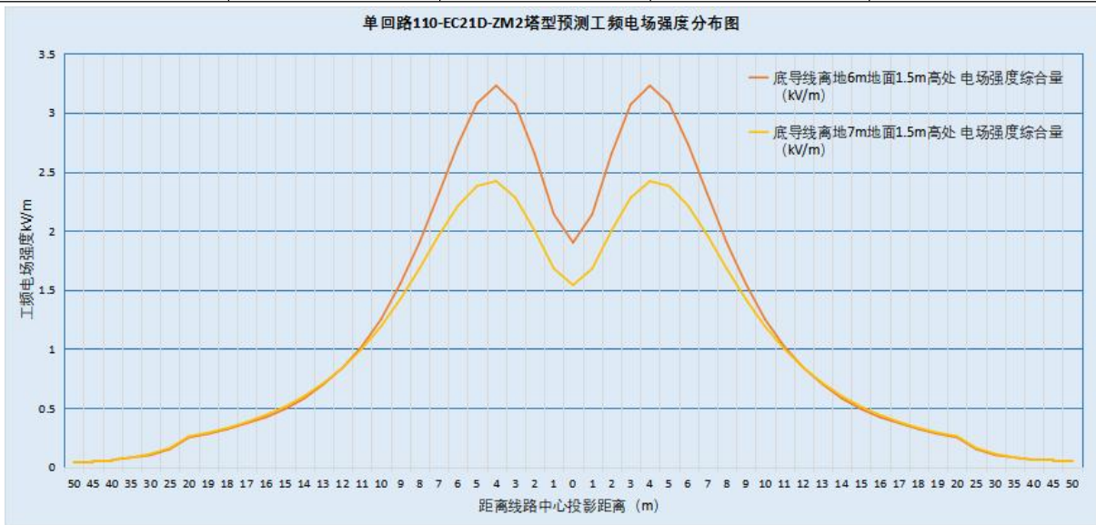
图 3-2 单回路 110-EC21D-ZM2 塔型工频电场强度分布图
