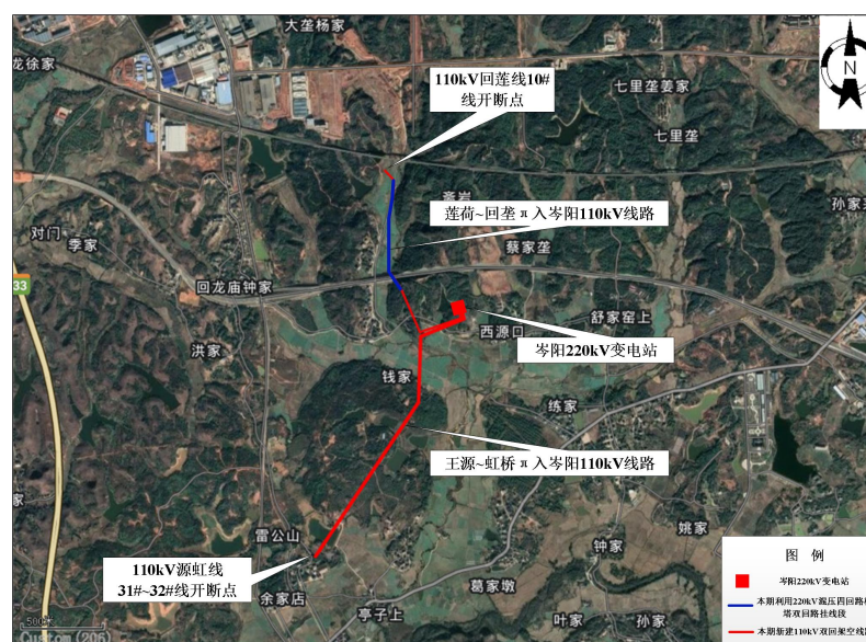
图 2-1 本工程 110kV 线路工程线路路径示意图
