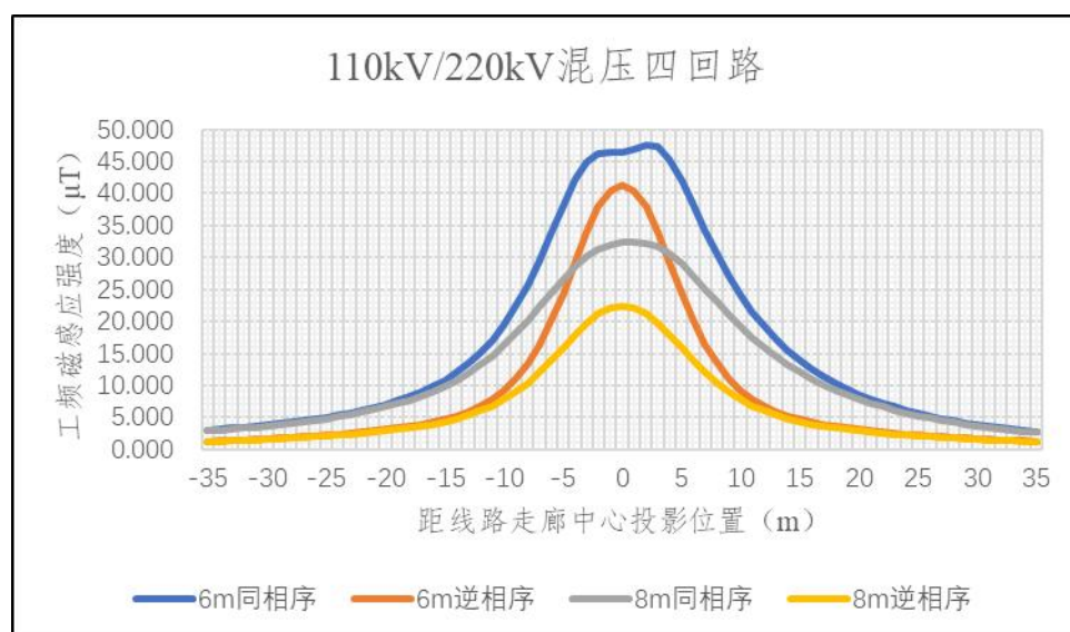
图 3-8 110kV/220kV 混压四回输电线路工频磁感应强度预测趋势图
