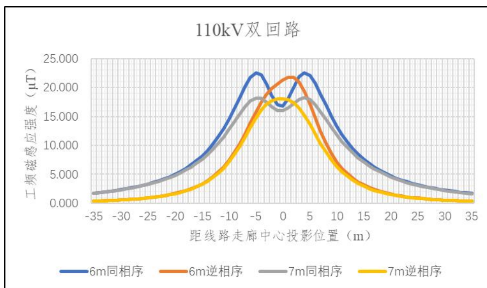
图 3-6 110kV 双回输电线路工频磁感应强度预测趋势图
