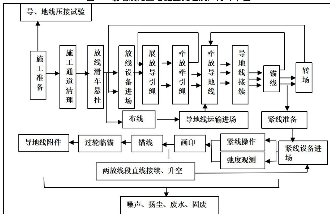
图2-3 架线施工流程图
