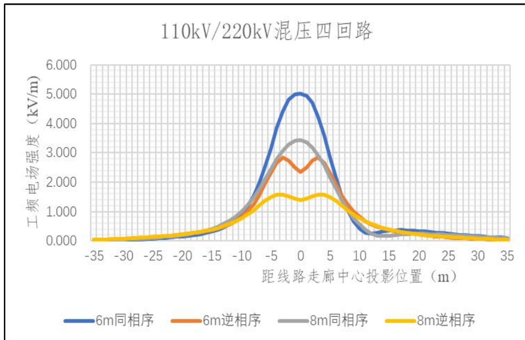
图 3-7 110kV/220kV 混压四回输电线路工频电场强度预测趋势图
