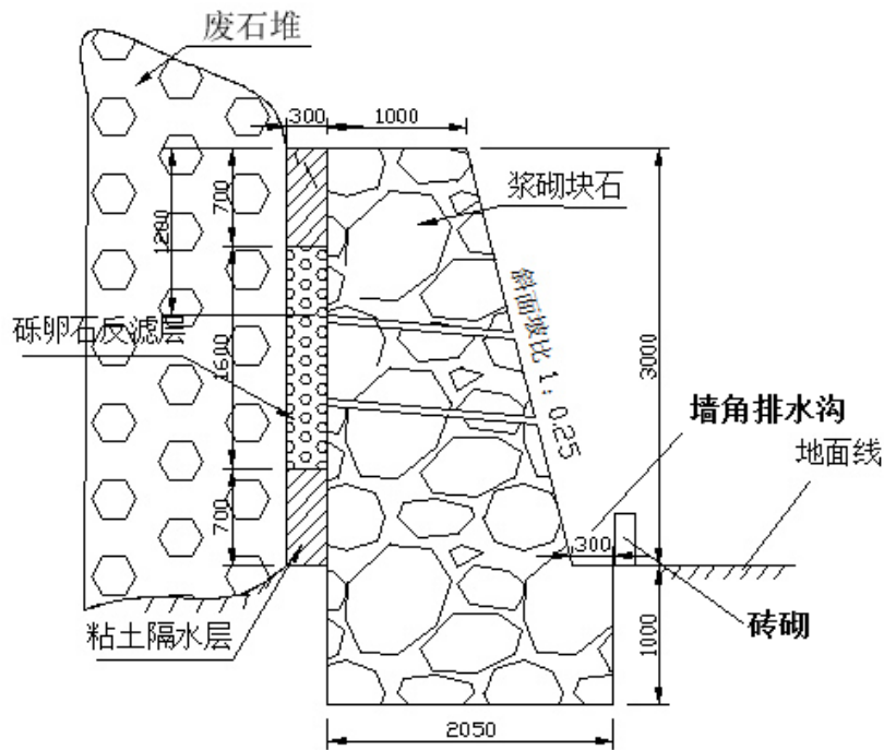
图 10-3 挡土墙设计图
