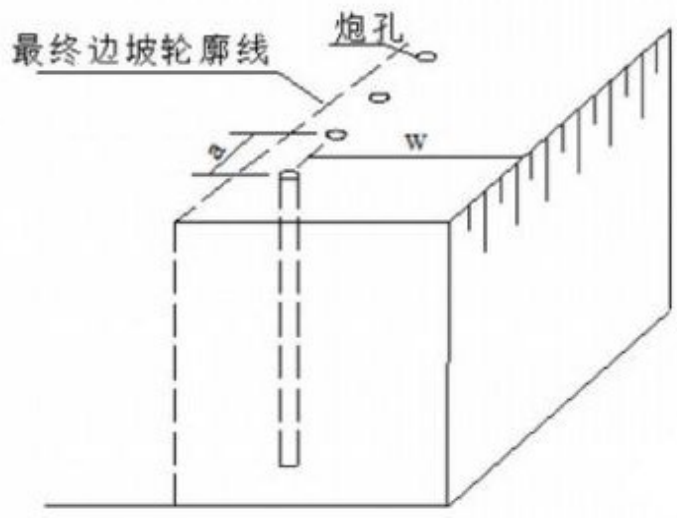
图 4-4 爆破示意图
