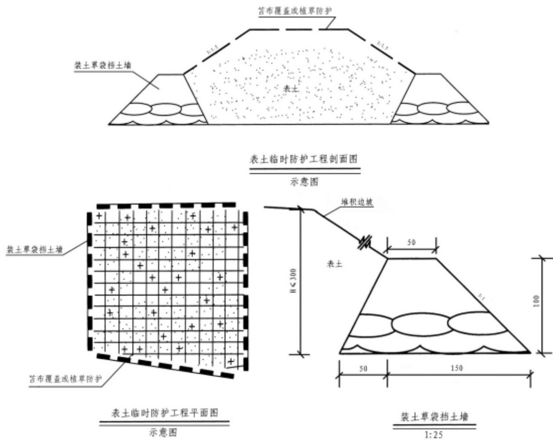
图 10-4 临时防护工程设计图
