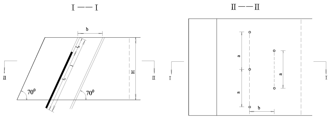
图 4-3 爆破参数图
