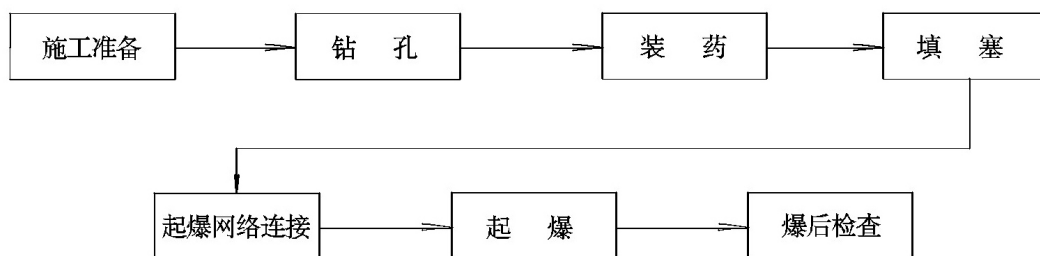
图 4-2 爆破施工工艺过程
