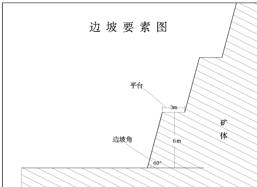
图 4-1 台阶参数示意剖面图
